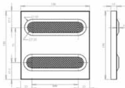
DIRECTIONAL TILE กระเบื้องพื้นผิวต่างสัมผัส ชนิดบอกทิศทาง
